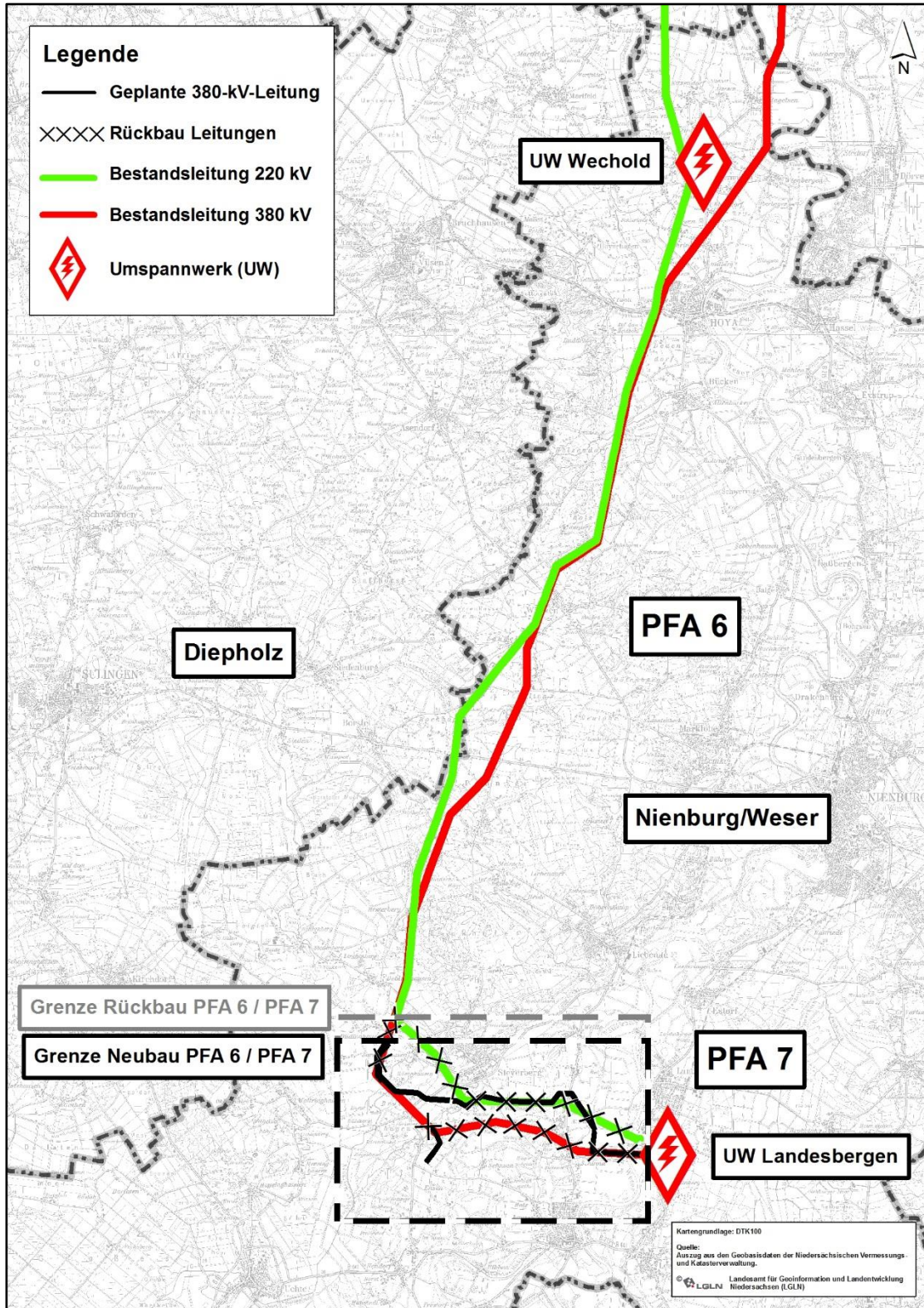
Abbildung 1: Lage der beantragten 380-kV-Leitung LH-10-3039, Rückbau der 220-kV-Leitung (LH-10-2010) und der 380-kV-Leitung (LH-10-3003) im Planfeststellungsabschnitt (PFA) 7
