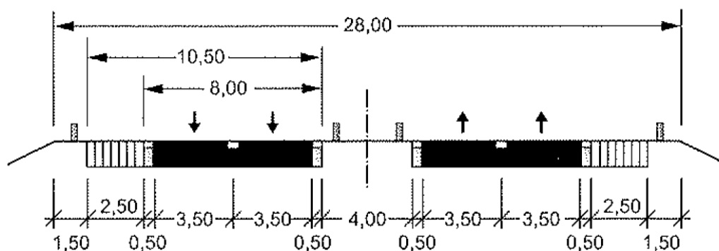
Abbildung 31: Regelquerschnitt RQ 28
