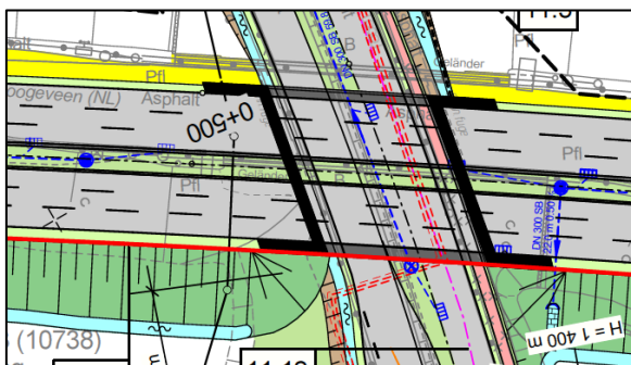
Abbildung 66: BW PA 1/20 - Ausschnitt Lageplan, U 5, Bl. 11
