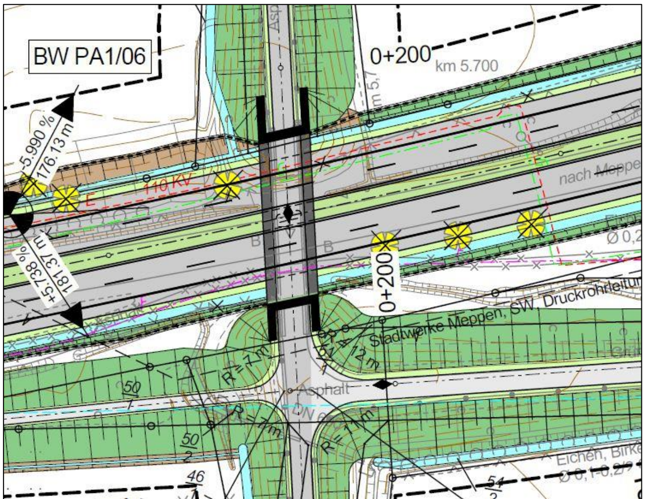
Abbildung 51: BW PA 1/06 - Ausschnitt Lageplan, U 5, Bl. 4
