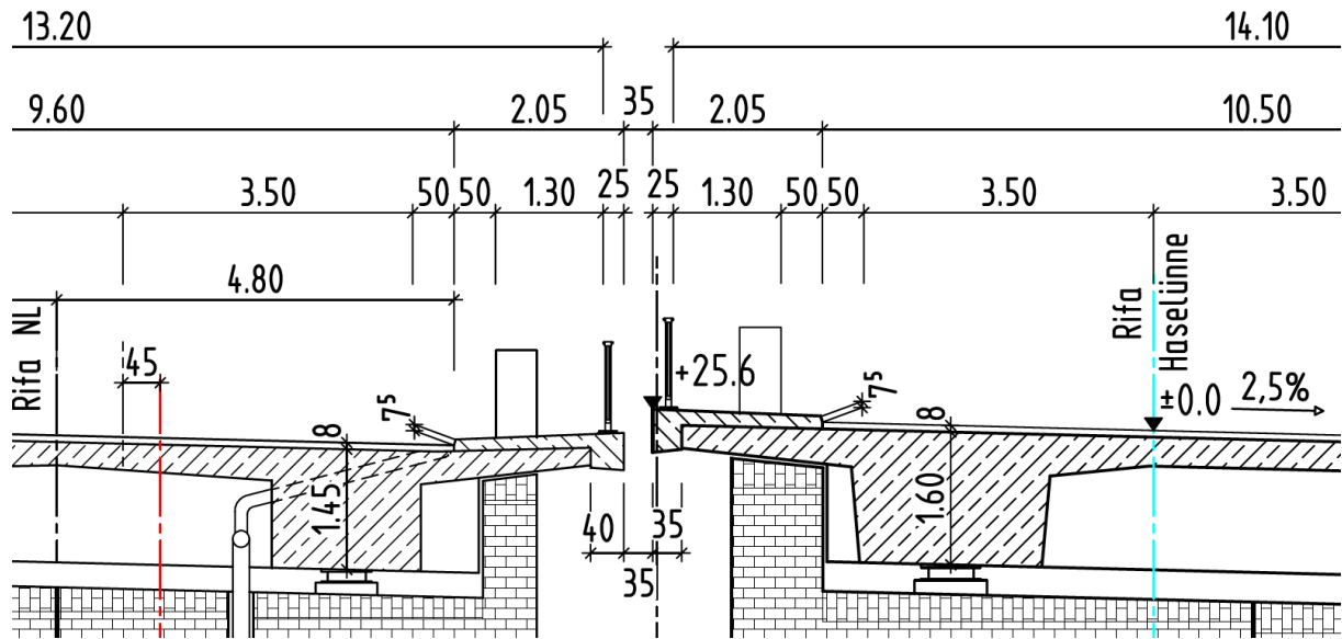
Abbildung 33: Bsp. Kappenausbildung BW 11 - Blick in Stationierungsrichtung
