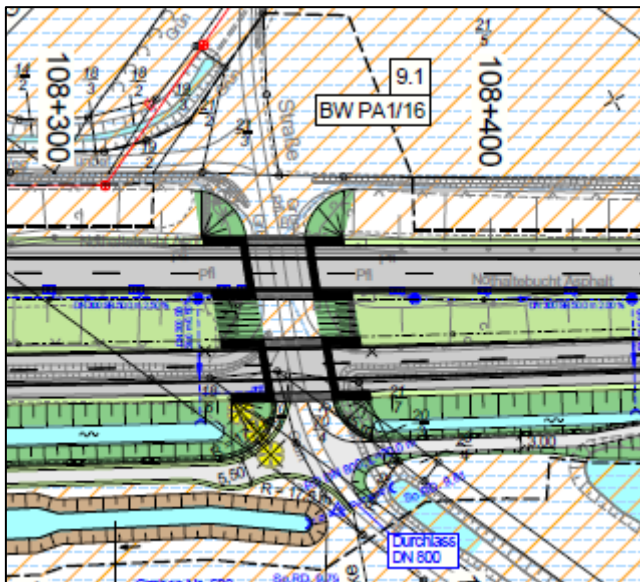
Abbildung 61: BW PA 1/16 - Ausschnitt Lageplan, U 5, Bl. 9
