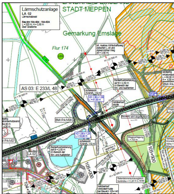
Abbildung 54: Bereich Abbemühlener Weg (Ausschnitt Übersichtslageplan U3, Bl. 2)
