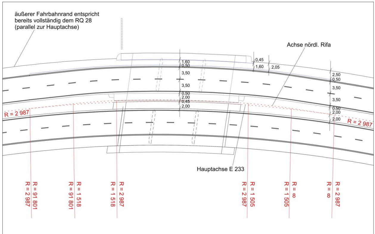
Abbildung 32: Systemskizze zur Achs- und Fahrplananordnung im Bereich der 3 BW über Flutmulde und Altarm
