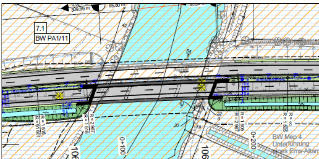
Abbildung 56: BW PA 1/11 - Ausschnitt Lageplan, U 5, Bl. 7
