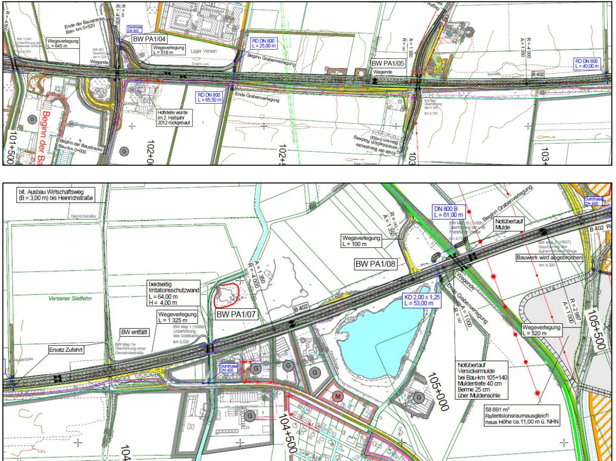
Abbildung 18: VGA 2A - Verbreiterung Nord – Nord (vgl. auch Anlage 3.3)
