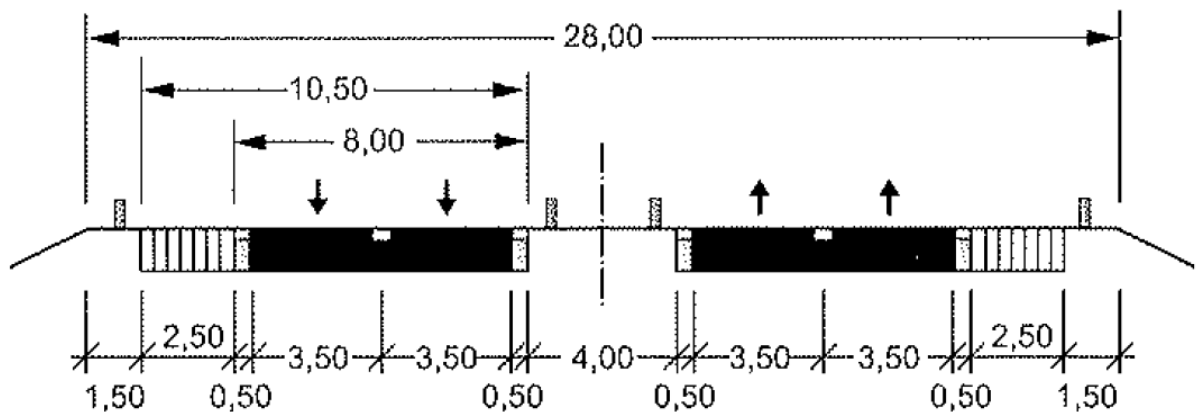
Abbildung 29: Regelquerschnitt RQ 28
