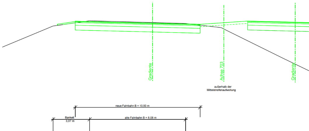
Abbildung 30: Beispielquerschnitt zur Fahrbahnanordnung im Bereich der Emsniederung
