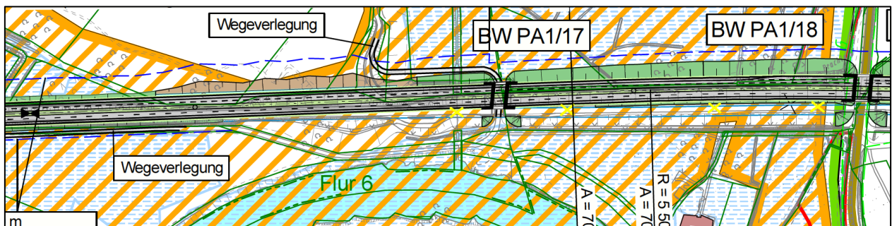
Abbildung 25: Borkener Berg - Verbreiterung nach Norden (Ausschnitt)
