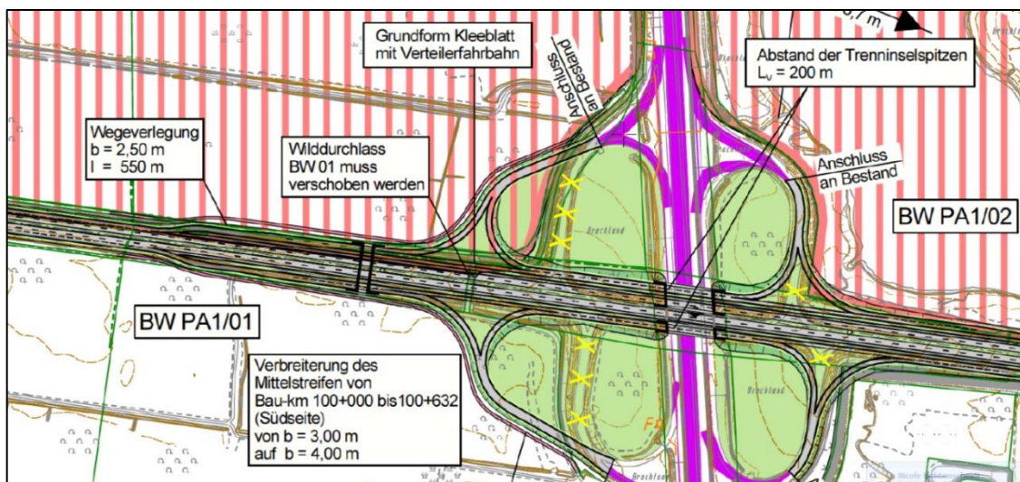
Abbildung 13: VGA 1 - Verbreiterung nach Norden (Ausschnitt)
