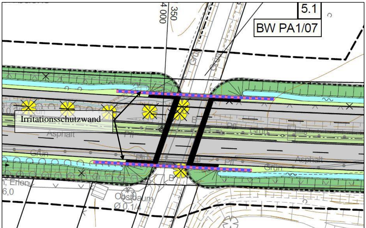
Abbildung 52: BW PA 1/07 - Ausschnitt Lageplan, U 5, Bl. 5
