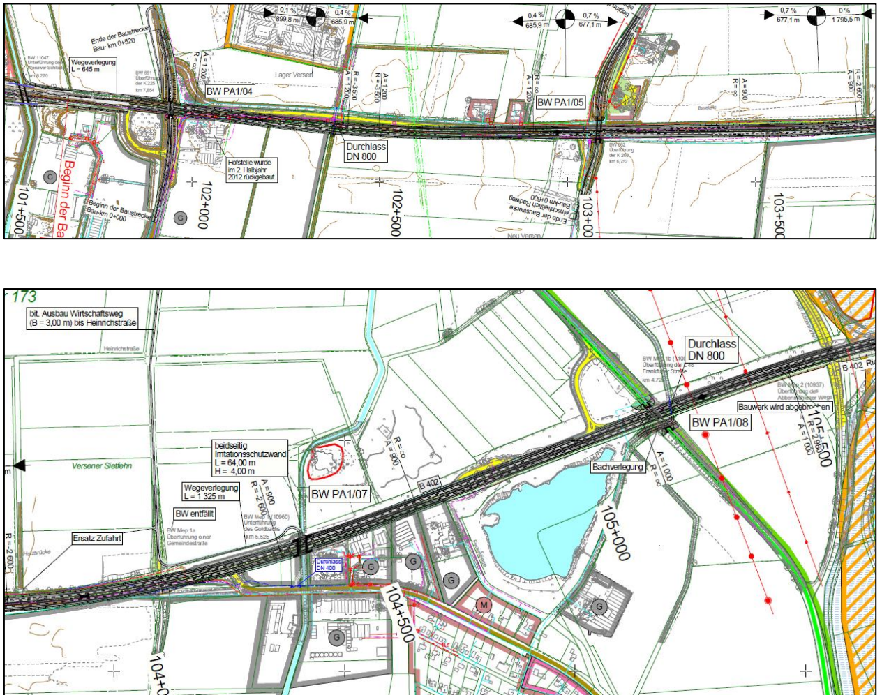
Abbildung 16: VGA 2A - Verbreiterung Süd (vgl. auch Anlage 3.1)
