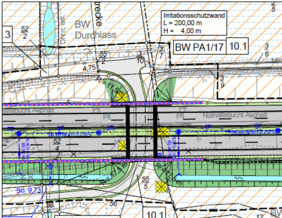
Abbildung 62: BW PA 1/17 - Ausschnitt Lageplan, U 5, Bl. 10
