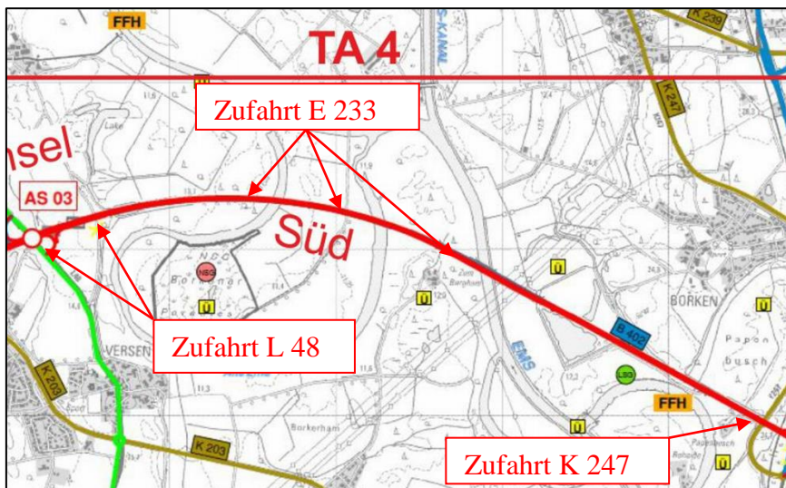
Abbildung 83: Baustellenzufahrt Emsniederung
