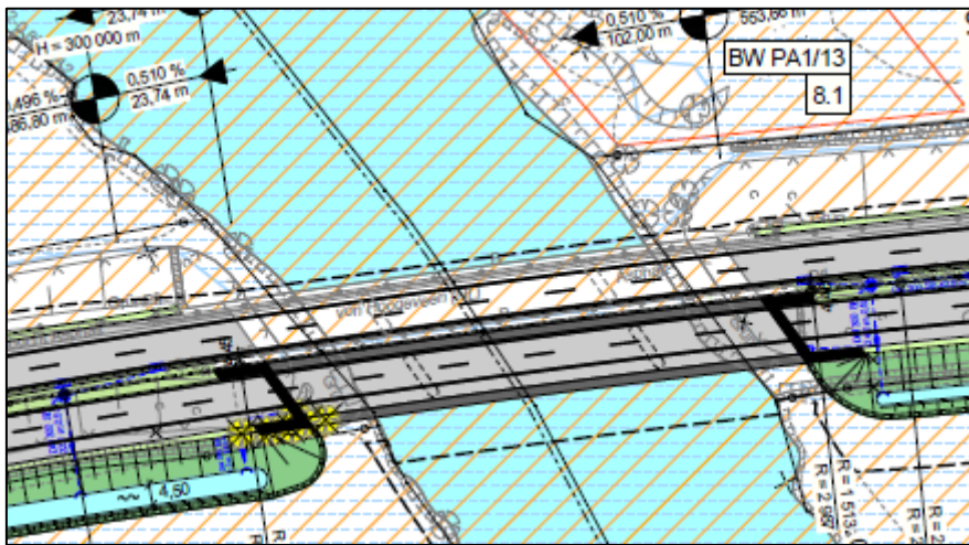
Abbildung 58: BW PA 1/13 - Ausschnitt Lageplan, U 5, Bl. 8
