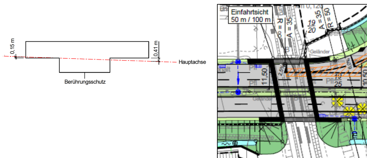
Abbildung 64: BW PA 1/19 - Systemdarstellung vorhandene südliche Kappe und Achslage, Ausschnitt Lageplan U 5, Bl. 11
