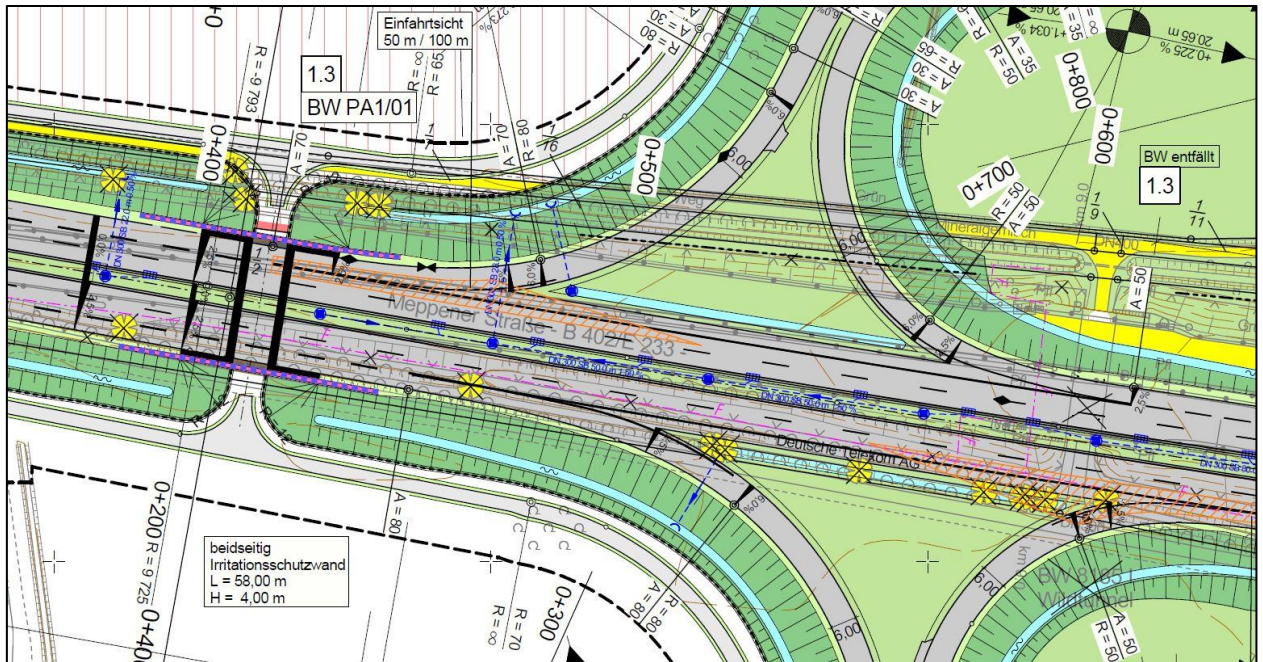
Abbildung 46: BW PA 1/01 - Ausschnitt Lageplan, U 5, Bl. 1
