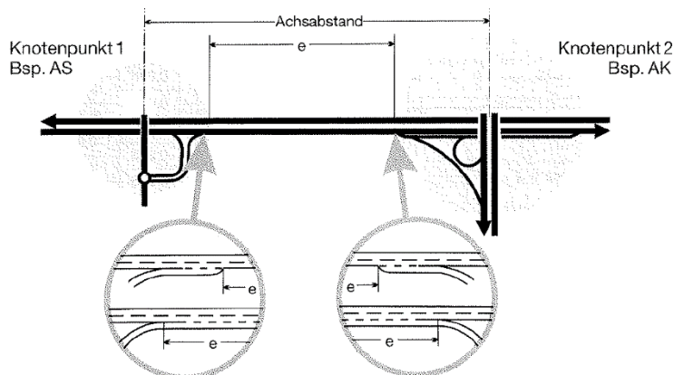
Abbildung 34: Systemskizze der RAA zu Knotenpunkten
