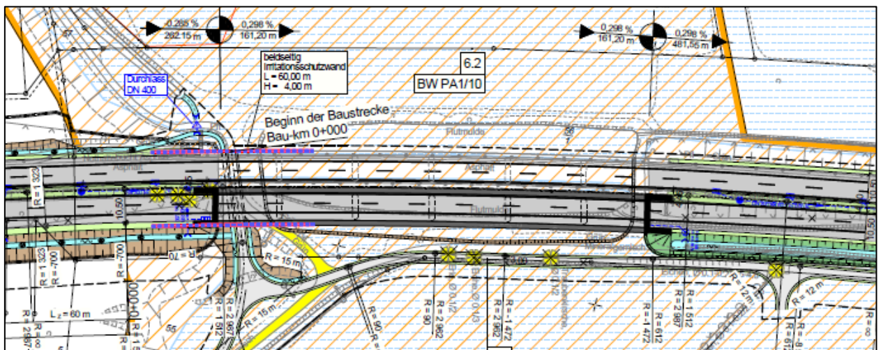
Abbildung 55: BW PA 1/10 - Ausschnitt Lageplan, U 5, Bl. 6
