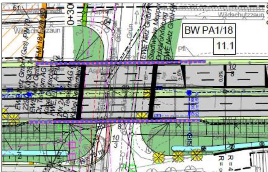
Abbildung 63: BW PA 1/18 - Ausschnitt Lageplan, U 5, Bl. 11
