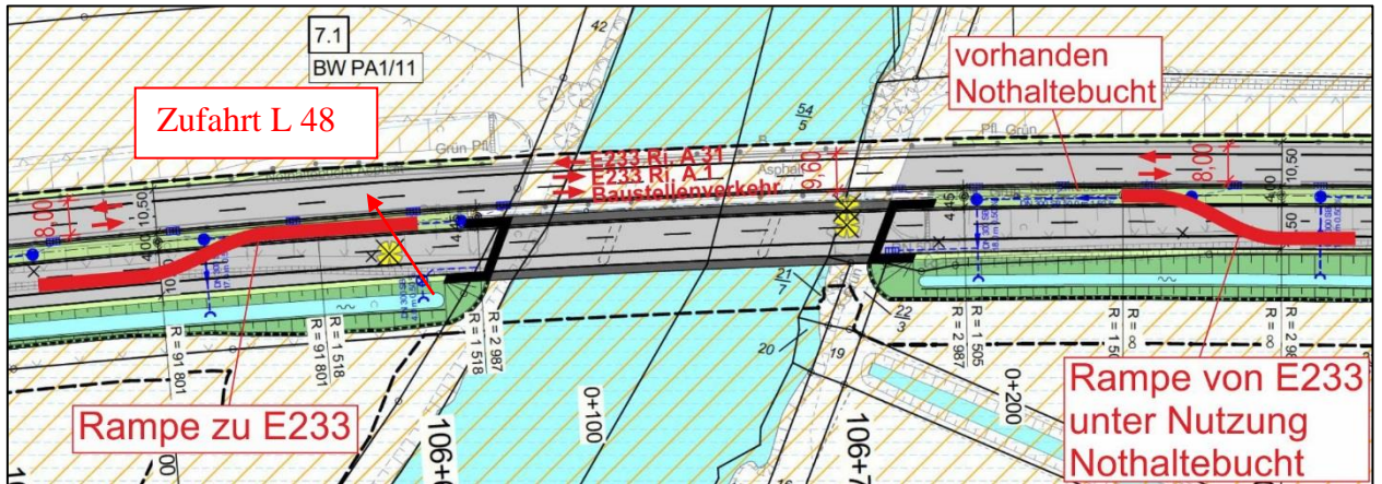
Abbildung 84: Prinzipdarstellung Rampen/BW Emsniederung
