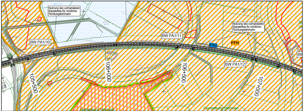
Abbildung 21: Borkener Paradies - Verbreiterung nach Süden (Ausschnitt)
