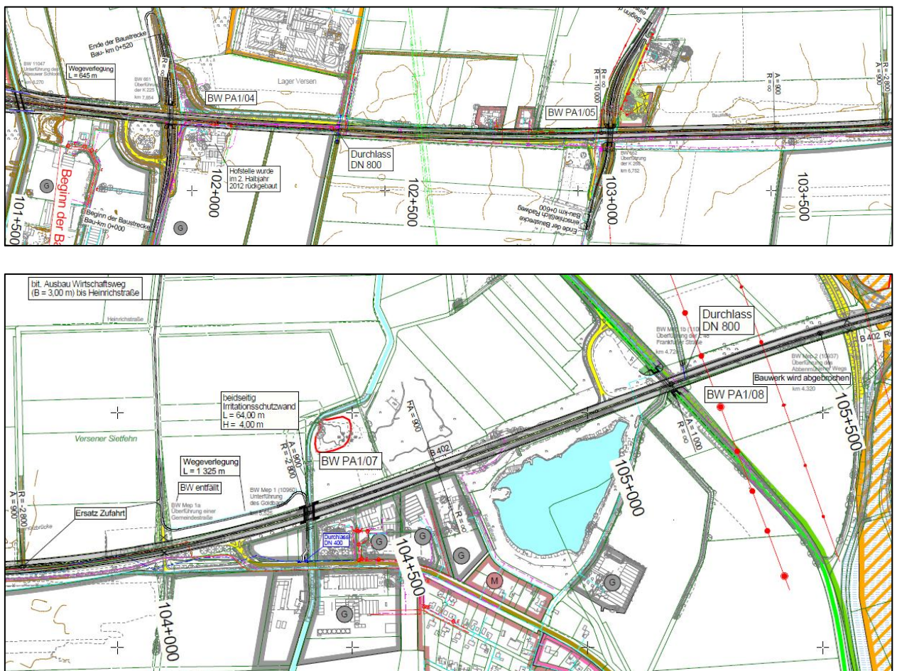
Abbildung 17: VGA 2A - Verbreiterung Nord (vgl. auch Anlage 3.2)
