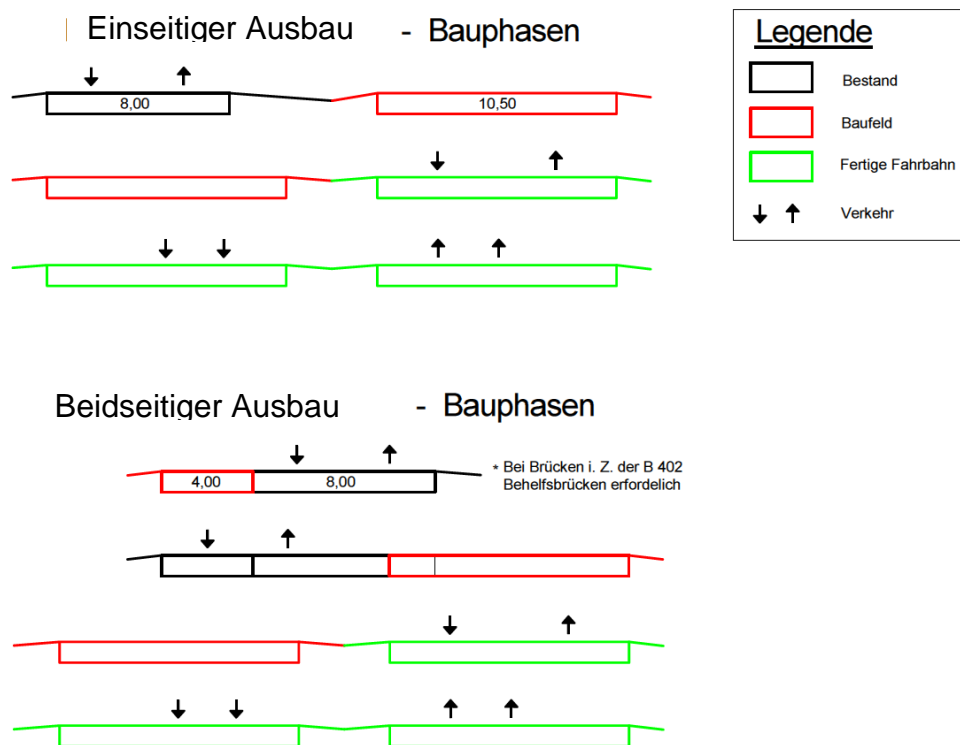
Abbildung 9: Schematischer Vergleich von Ausbaumöglichkeiten
