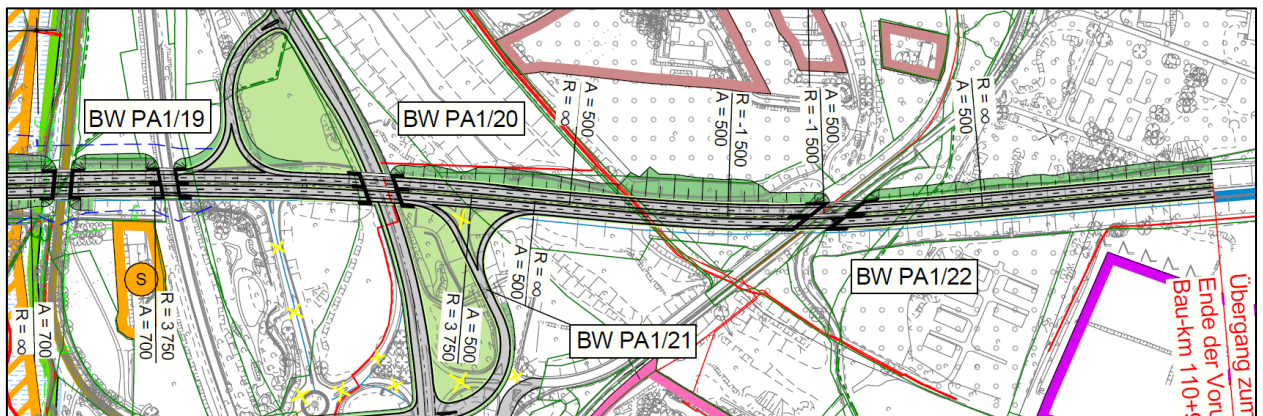
Abbildung 28: VGA 3B - Wechsel der Ausbauseite von Süd nach Nord
