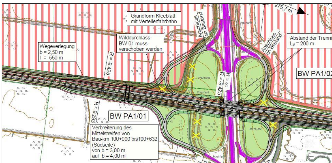
Abbildung 14: VGA 1 - Verbreiterung nach Süden (Ausschnitt)
