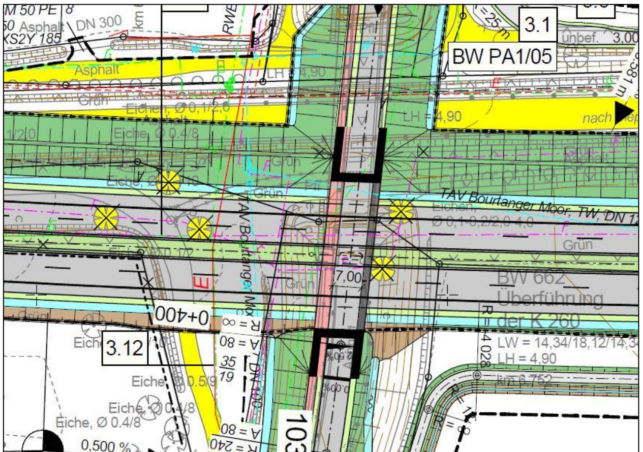
Abbildung 50: BW PA 1/05 - Ausschnitt Lageplan, U 5, Bl. 3
