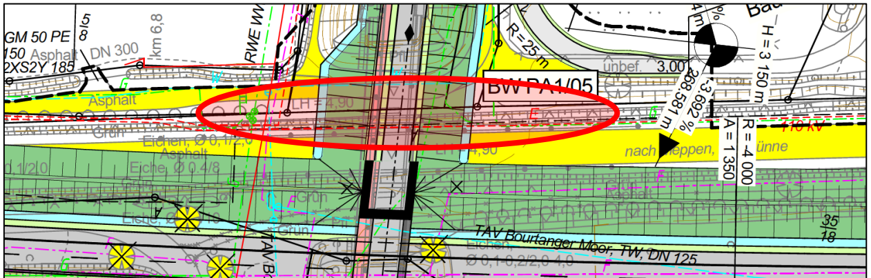
Abbildung 80: Bereich Neuversener Straße - Provisorium für E 233
