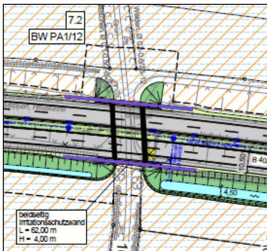
Abbildung 57: BW PA 1/12 -Ausschnitt Lageplan, U 5, Bl. 7
