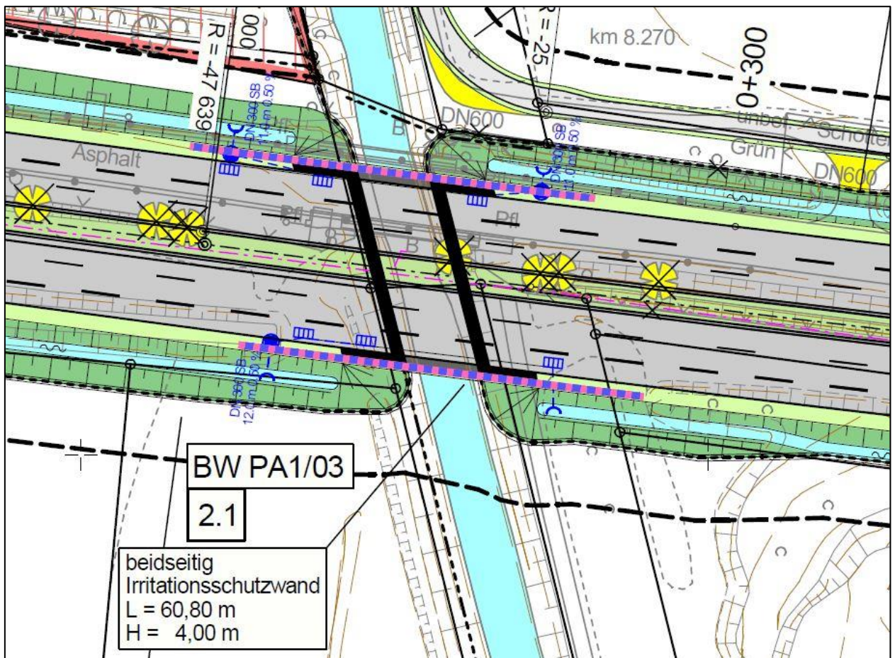
Abbildung 48: BW PA 1/03 - Ausschnitt Lageplan, U 5, Bl. 2
